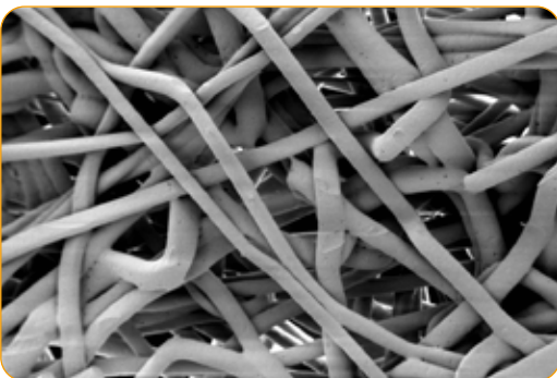
Struttura interna cartuccia / Internal structure of the cartridge (100 μm)
